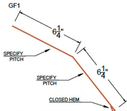
GAMBREL
