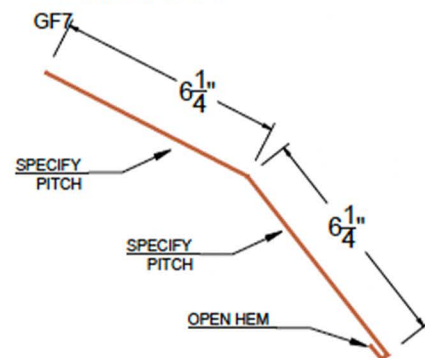
GAMBREL
