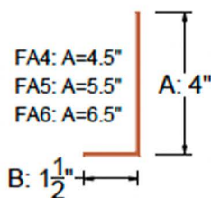
FASCIA FA4, FA5, FA6
